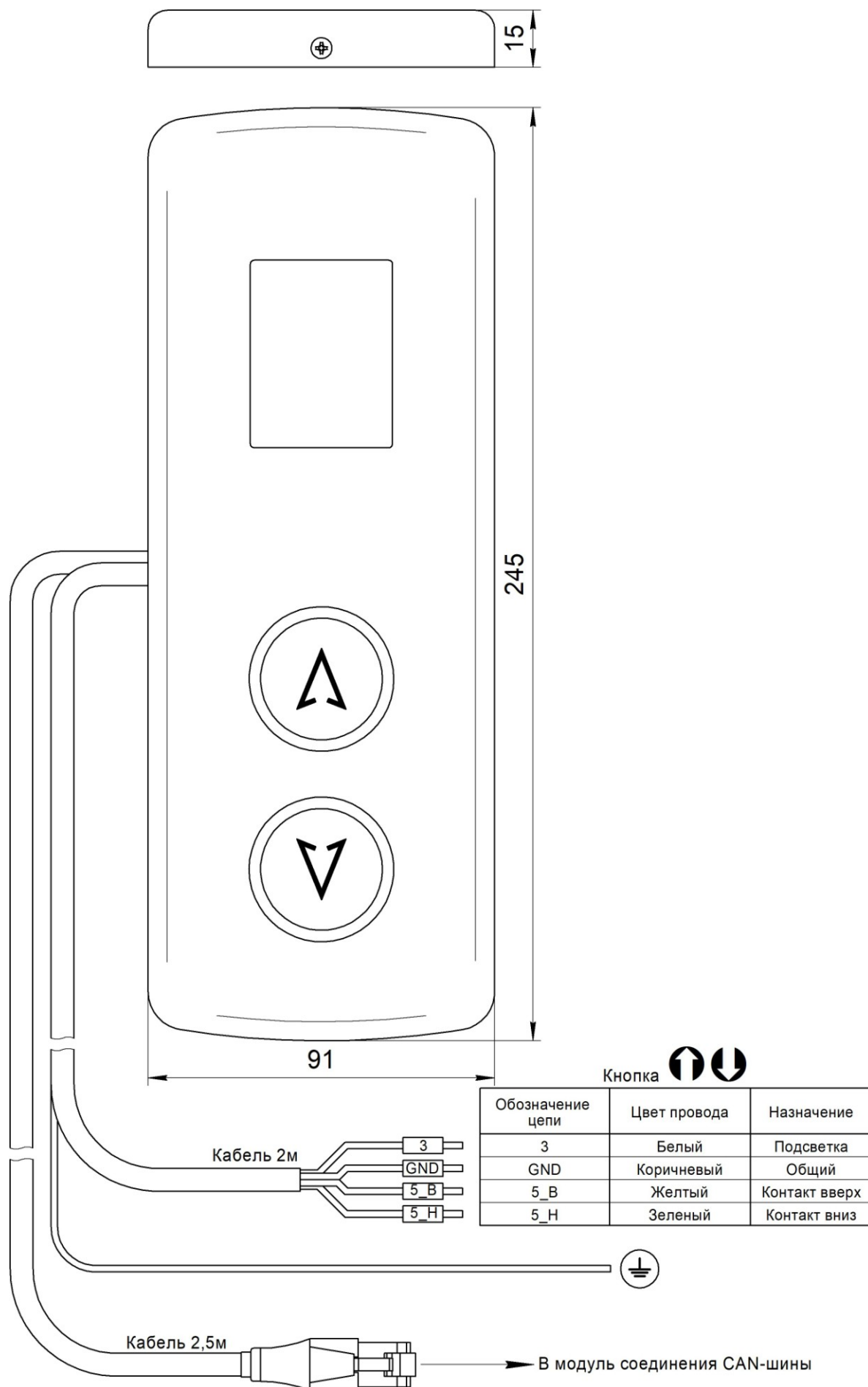
Рис.1 Внешний вид, габаритные и установочные размеры Вызывного поста ЦИРКОН (жгут RJ45) НШЕК.468381.021
